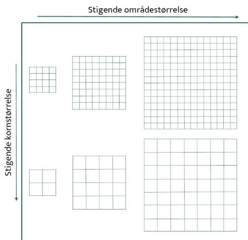
Figur 7: En kvadrat-sampling kan se meget forskellig ud afhængig af hvilken områdestørrelse og kornstørrelse, man arbejder med.
