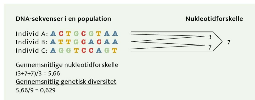
Figur 6: Sådan kan man måle genetisk diversitet. I dette eksempel kigger man på DNA-sekvenser fra tre individer. Alle DNA-sekvenserne har en længde på 9 nukleotider. Der er 3 nukleotidforskelle mellem individ A og B, 7 nukleotidforskelle mellem individ B og C og 7 nukleotidforskelle mellem individ A og C. Gennemsnittet af nukleotidforskelle mellem de tre individers DNA-sekvenser er altså (3+7+7)/3 = 5,66 nukleotider. Den gennemsnitlige genetiske diversitet for de tre individer finder man ved at dividere gennemsnittet af nukleotidforskelle med DNA-sekvensernes længde, altså 5,66/9 = 0,629 .
